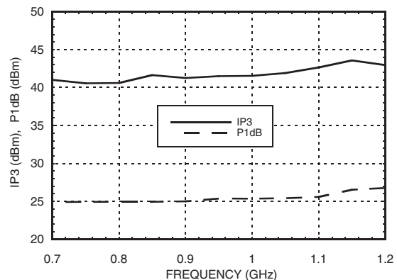
Output IP3 & P1dB
