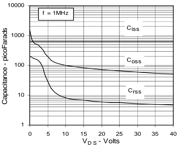
Fig. 11. Capacitance
