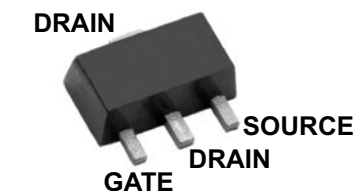
TO-243AA (SOT-89) (N8)
