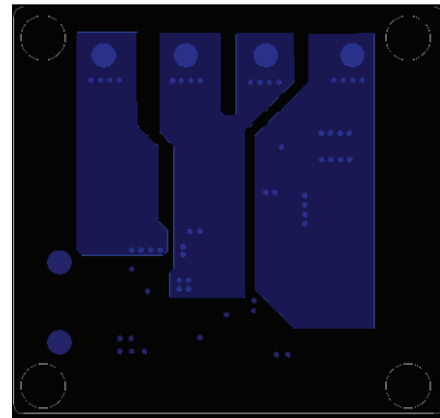
Fig. 27 - Bottom Layer
