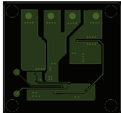
Fig. 28 - Inner Layer2
